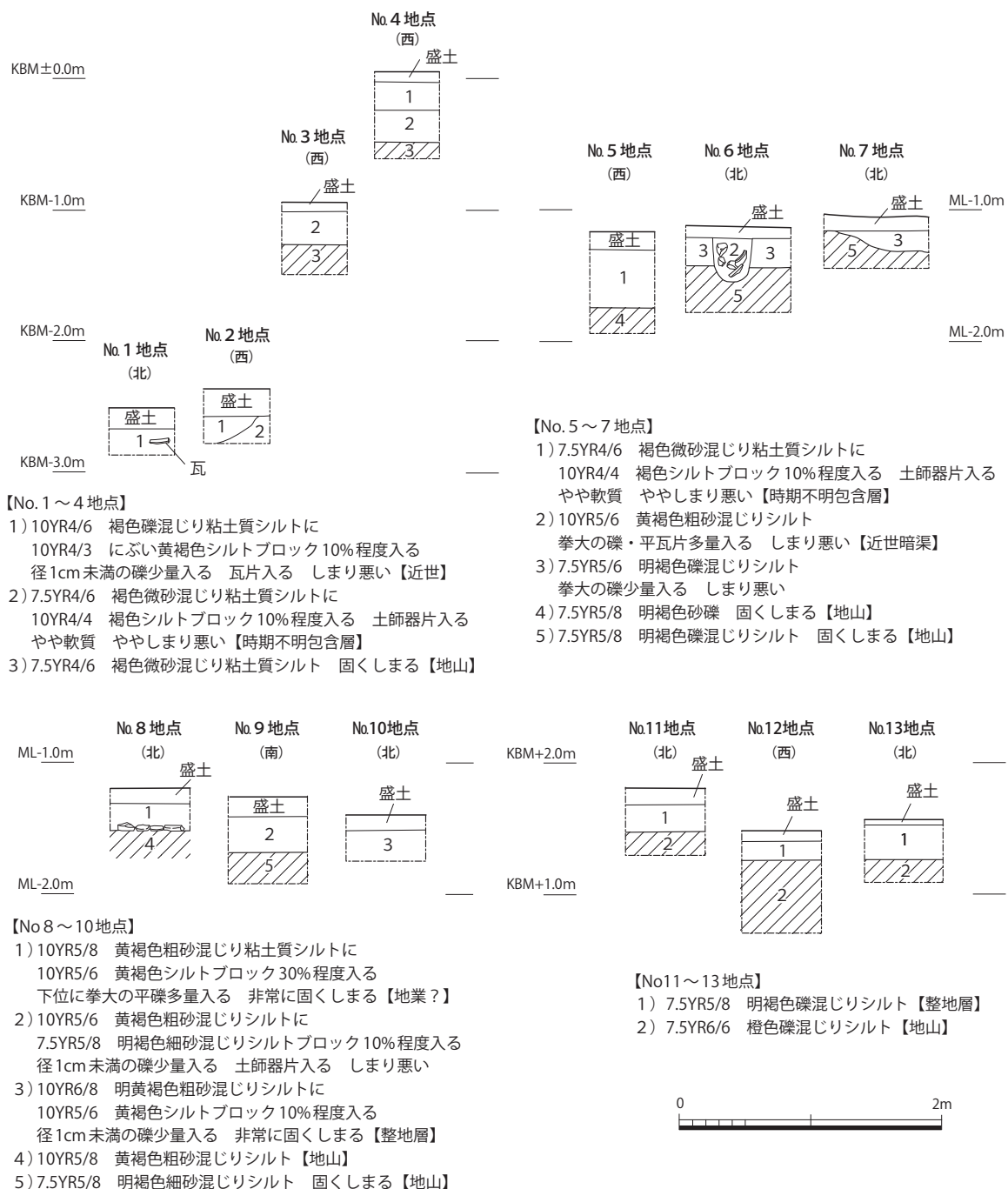
図50 No.1～13地点断面図（1：50）
