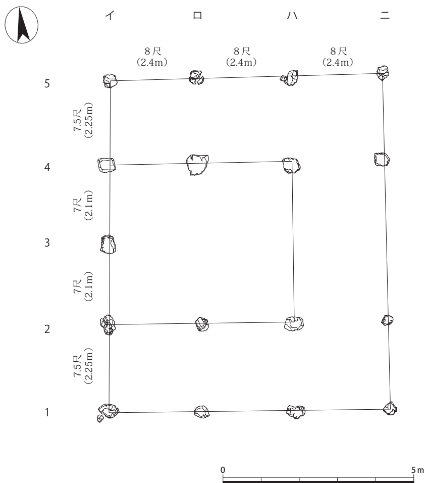
図 71 礎石建物平面図（1：100）
