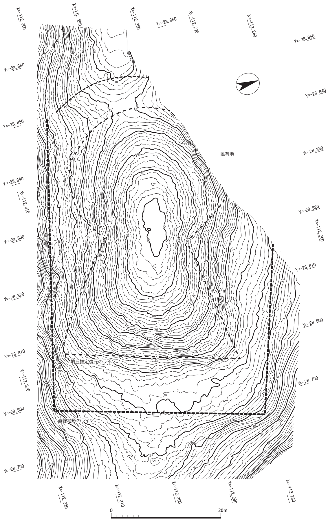
図 66 山田桜谷 1 号墳測量図 (1 : 400)
