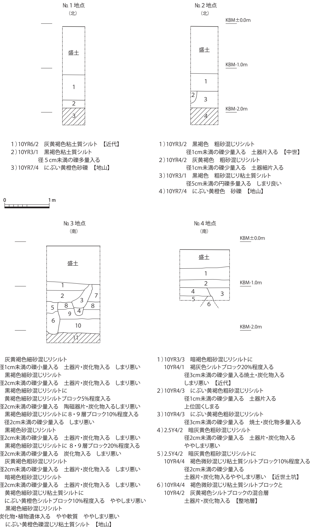
図8 No.1～4地点断面図(1:50)
