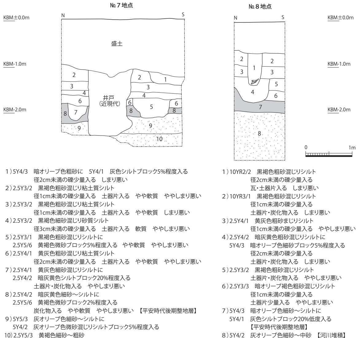
図27 No.7・8地点断面図（1：50）
