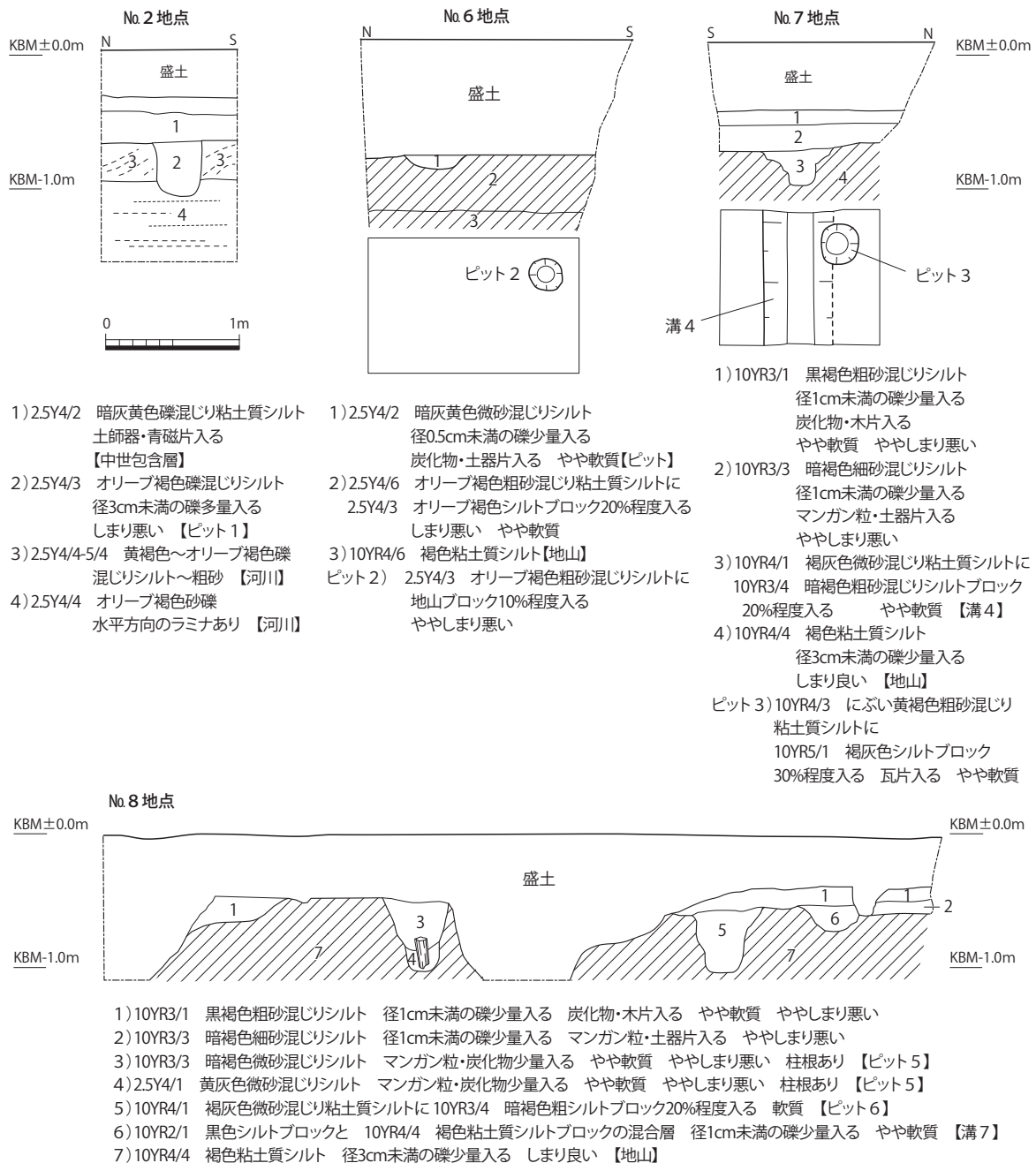
図31 No.2・8地点断面及びNo.6・7地点平・断面図（1：50）
