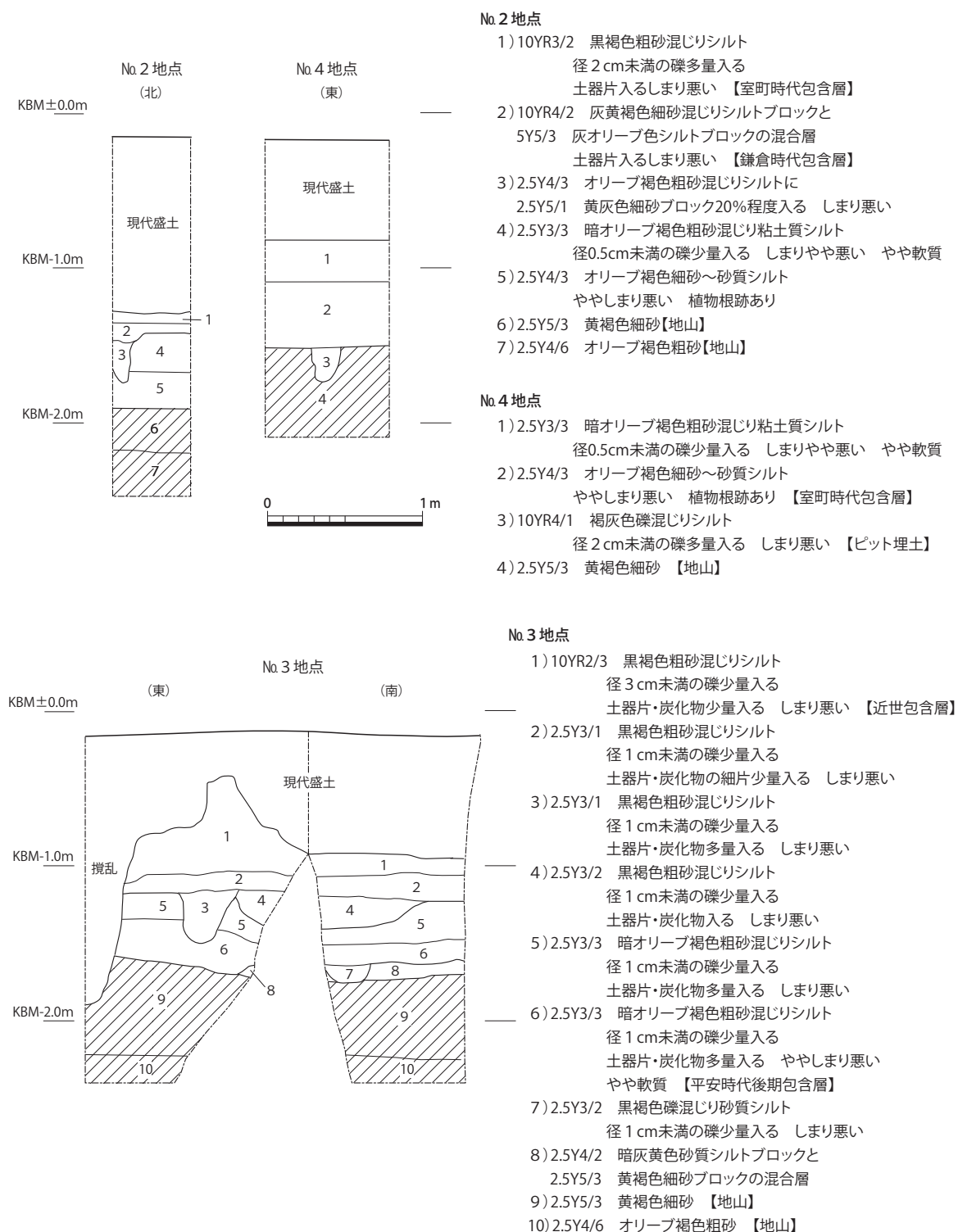
図 22 No. 2 ～ 4 地点断面図 (1 : 40)
